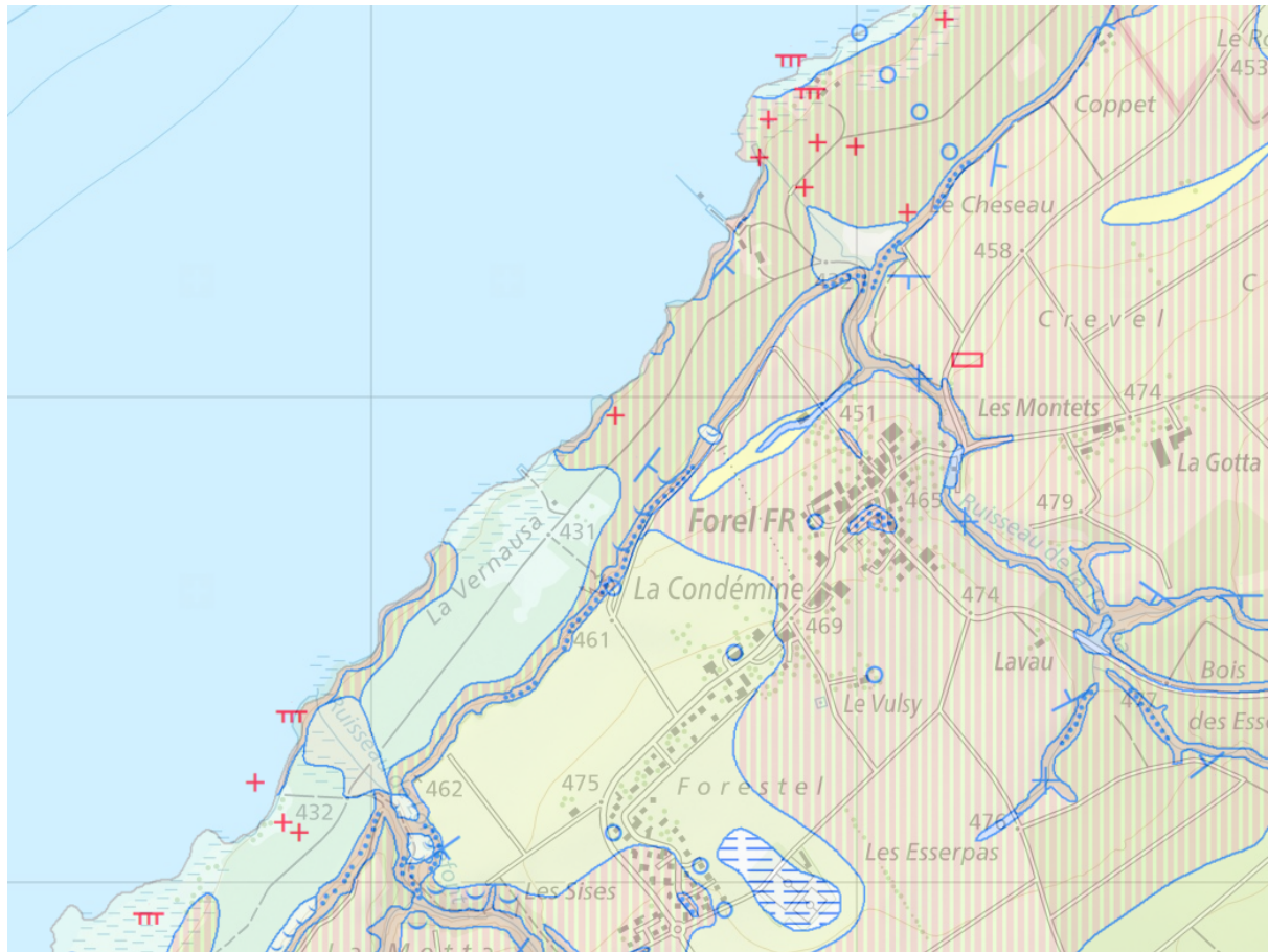
Abbildung 2. Geologische Karte der Umgebung Forel (aus Geologiekarten Geoportal Swisstopo; map.geo.admin.ch)
